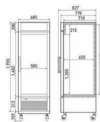
TGF-23SD(B) • Мощность, кВт: 0,49
