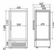
TGF-10SD(W) • Мощность, кВт: 0,37
