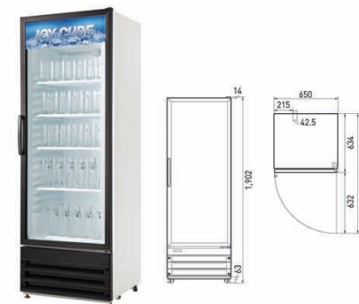
FRS-505CF • Мощность, кВт: 0,245 • Объем, л : 420 • Температурный режим : -5° ~ +3° • Кол-во полок : 4 • Вес, кг : 80 • Габариты, ш/г/в (мм) : 650x634x1902
