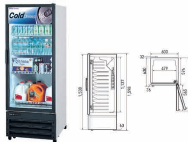
FRS-300RP • Мощность, кВт: 0,185 • Объем, л : 269 • Температурный режим : 0° ~ +8° • Кол-во полок : 4 • Вес, кг : 76 • Габариты, ш/г/в (мм) : 600x594x1598
