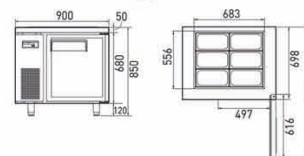
ВИД СБОКУ
