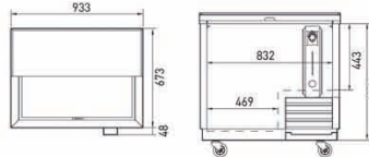
TBC-36SD / TBC-36SB • Мощность, кВт: 0,185
