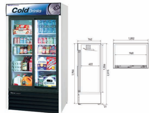
FRS-1000R • Мощность, кВт: 0,37 • Объем, л : 951 • Температурный режим : 0° ~ +8° • Кол-во полок : 8 • Вес, кг : 192 • Габариты, ш/г/в (мм) : 1052x762x2015
