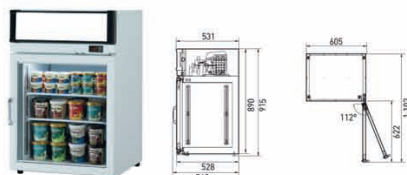
FS-120F • Мощность, кВт: 0,245
