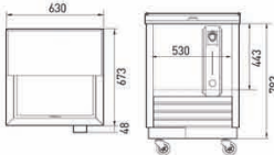
TBC-24SD / TBC-24SB • Мощность, кВт: 0,075
