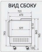
TBC-24SD / TBC-24SB • Мощность, кВт: 0,075
