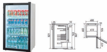
FRS-140R • Мощность, кВт: 0,075 • Объем, л : 123 • Температурный режим : 0° ~ +8° • Кол-во полок : 4 • Вес, кг : 34 • Габариты, ш/г/в (мм) : 480x526x867
