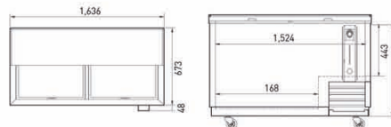
TBC-65SD / TBC-65SB • Мощность, кВт: 0,245
